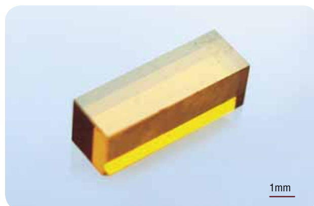
Элементы рентгеновской оптики из монокристаллов синтетического алмаза
